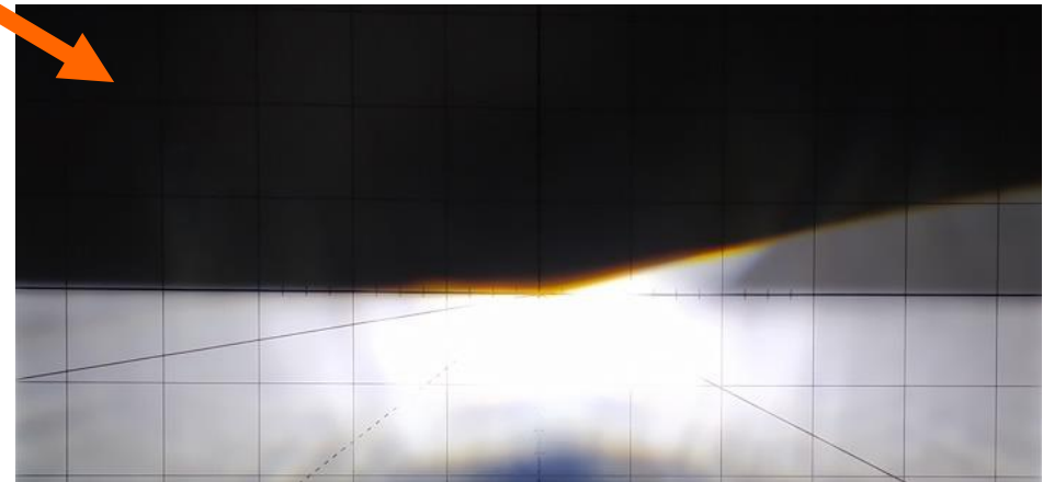
LEDDriving® HL INTENSE H7/H18 0° (стандартно положение)
